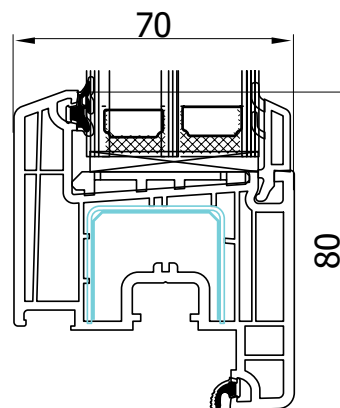
Flügelprofil
