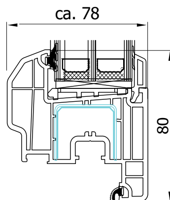
Flügelprofil
